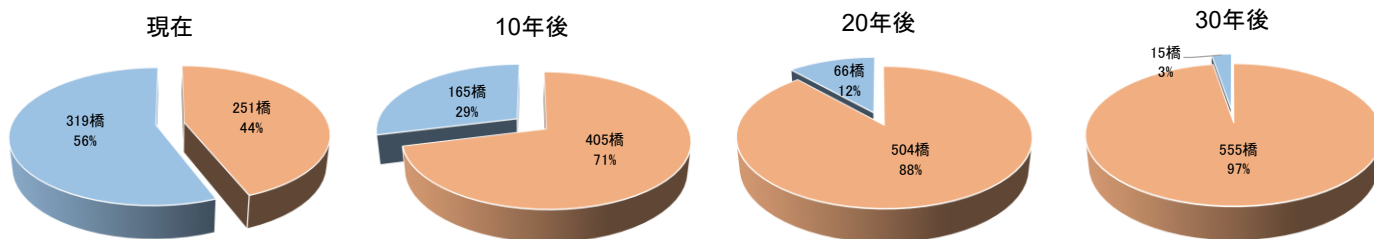
建設後 50 年を超す橋梁の割合
